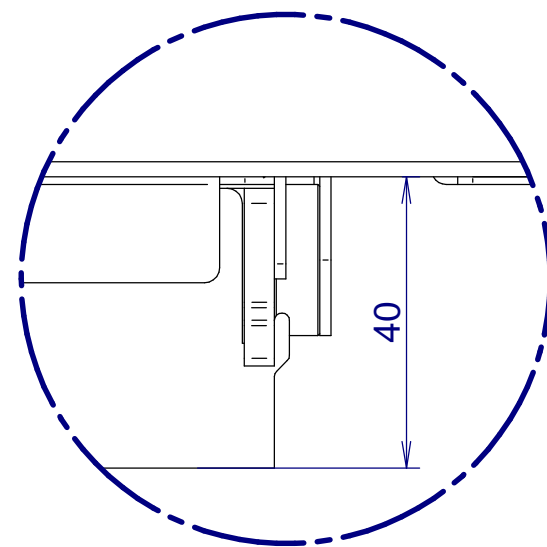
DETAIL A 1:1
